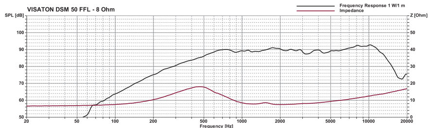
VISATON DSM 50 FFL - 8 Ohm
