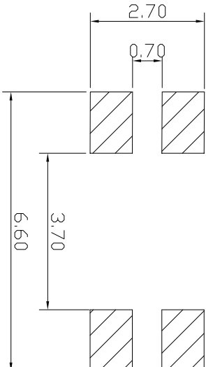
P.C.B LAYOUT
